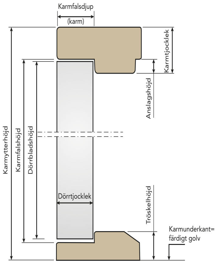
Vänsterhängd dörr
