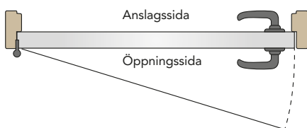
Vänsterhängd dörr
